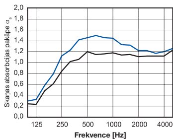
Perforēts alumīnija skārds ar kvadrātiskiem caurumiem QL 5/8 ar perforējuma laukumu 39,1 %
