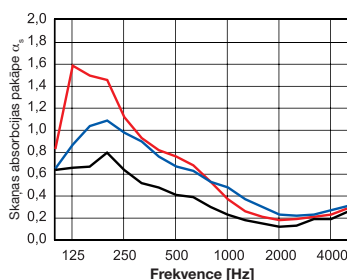
Neperforēts alumīnija skārds d = 1,5 mm
