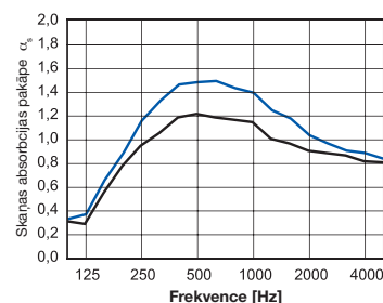
Perforēts alumīnija skārds ar apaļiem caurumiem RL 2.5/8.0 ar perforējuma laukumu 7,6 %
