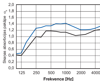
OWAcoustic® plātne ar uzlīmētu flīsu un Creaprint apdrucku
