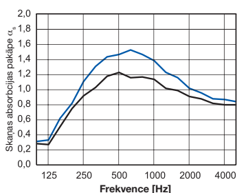
HDF/MDF plātne ar kvadrātisku perforējumu QP 10/22,5 ar perforējuma laukumu 20,7 %
